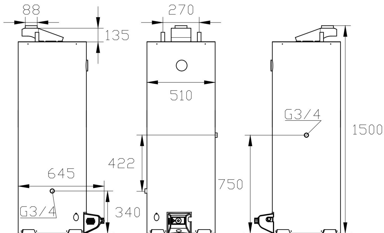
Рис. 6 Габаритные и присоединительные размеры НГВ ТЕПЛОПУС 150 л
