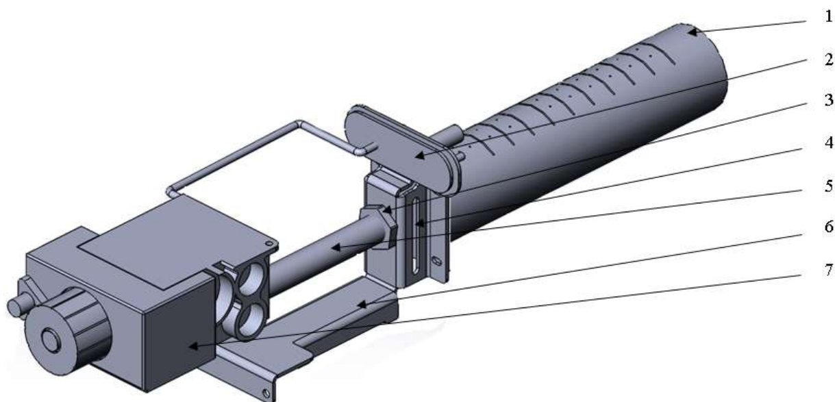
1 - Трубчатая горелка, 2 - Пилотная горелка, 3 - Переходник, 4 - Жиклер, 5 - Топливная рампа, 6 - Кронштейн ГГУ, 7 - Клапан газовый.
