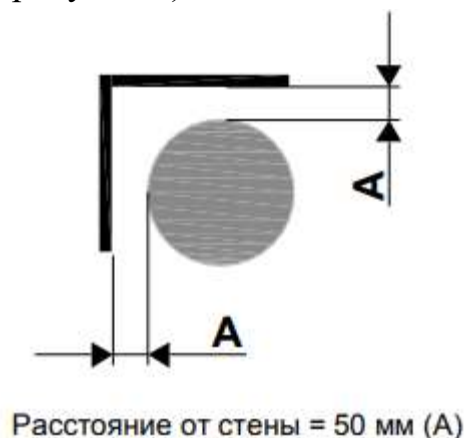
Рис.8 Размещение накопительного газового нагревателя в помещении
