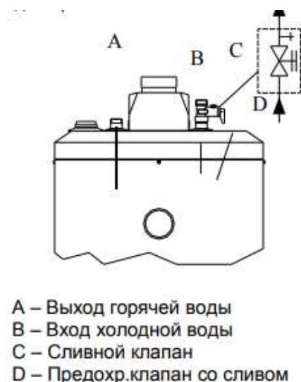
Рис. 11 Гидравлические подключения
