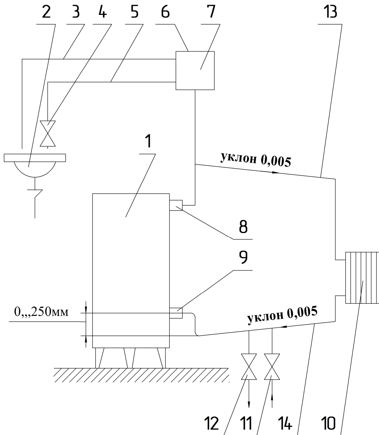
Рис.7 Схема присоединения аппарата к системе отопления
