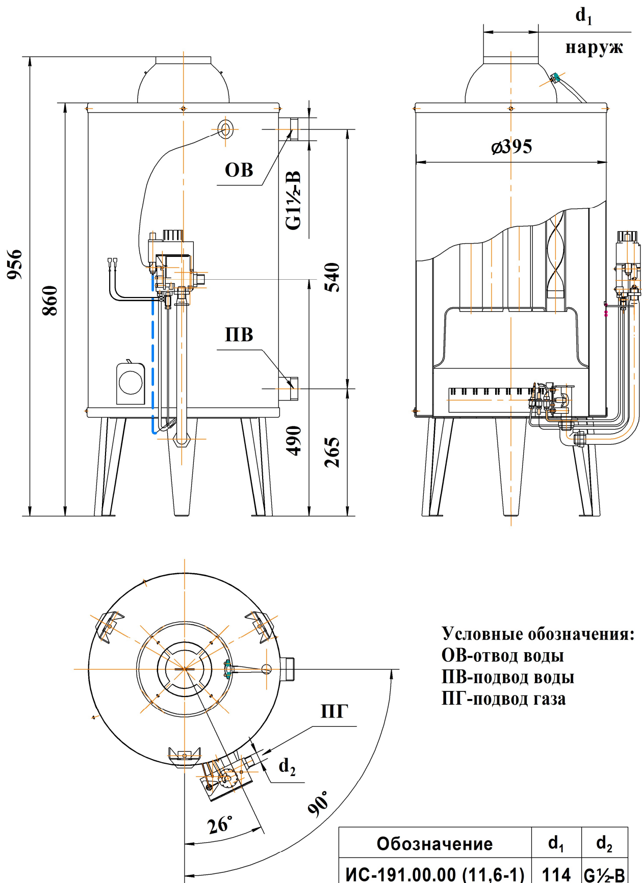
Рис.2 Габаритные и присоединительные размеры аппаратов АОГВ-11,6; 17,4
