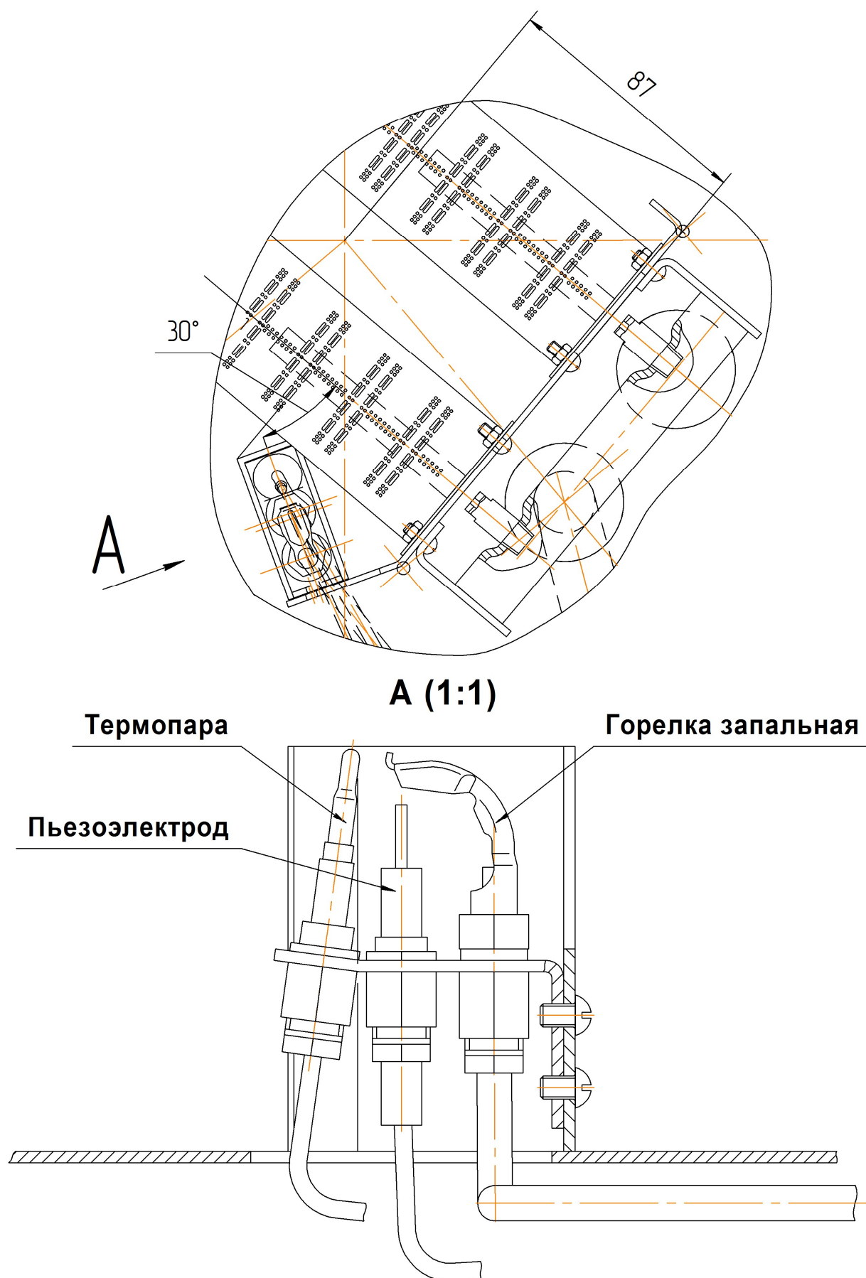
Рис.8а Схема расположения горелки основной и запальной для АОГВ-17,4
