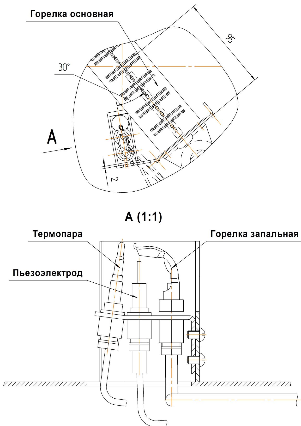
Рис.8 Схема расположения горелки основной и запальной для АОГВ-11,6
