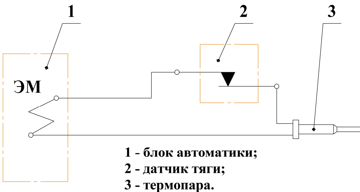
Рис.3 Схема электрическая
