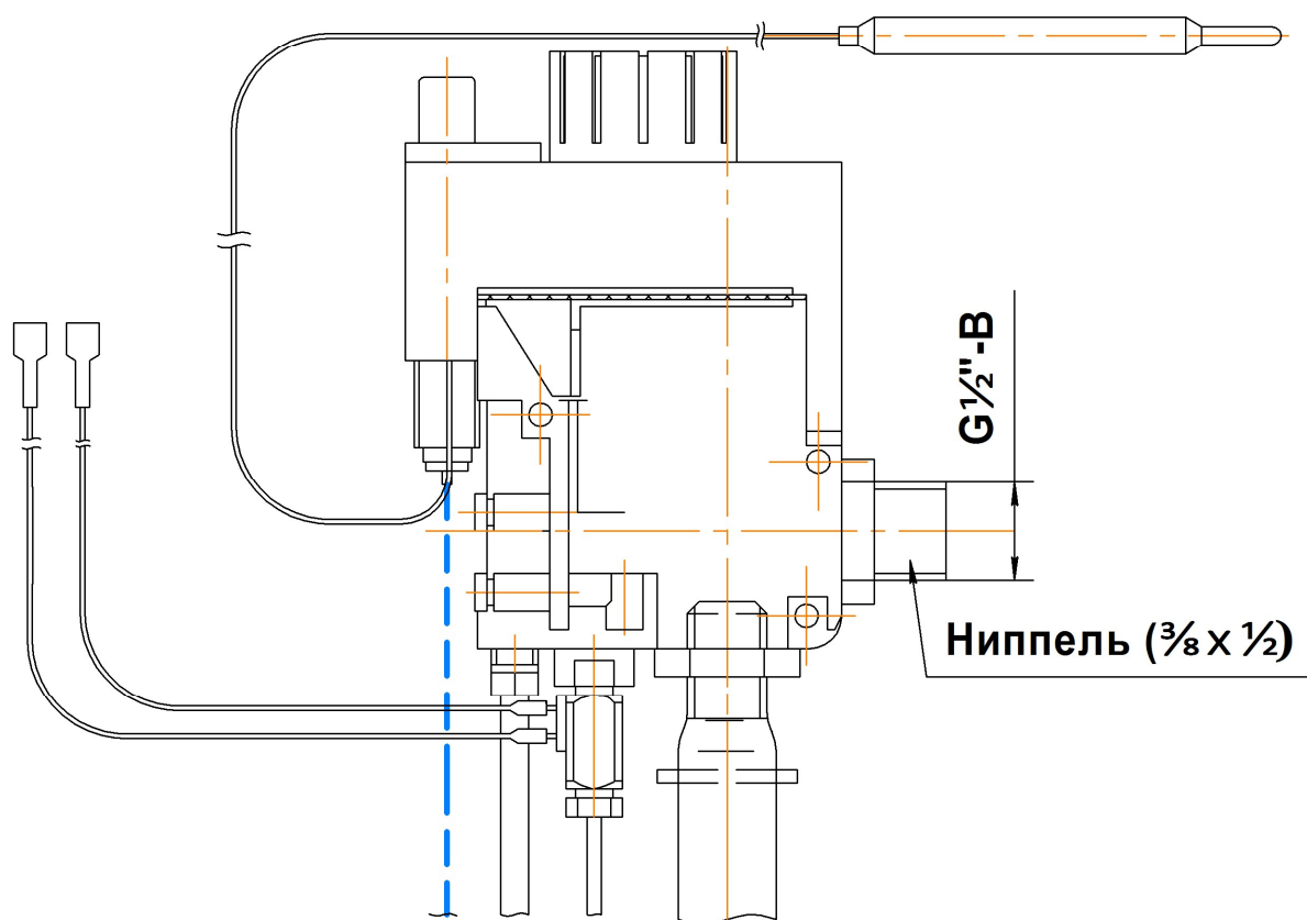
Рис.9 Подсоединение автоматики: для АОГВ-11,6-1
